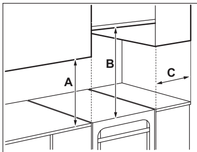
Minimális távolságok
