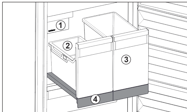
Fig. 32 Kihúzható rács IceTower egységgel
