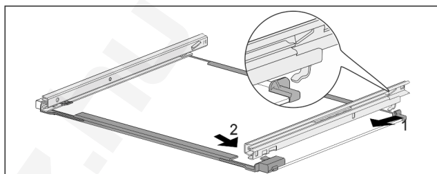
Fig. 51 Üveglap sínekkel
