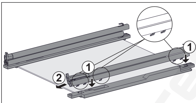
Fig. 63 Üveglap sínekkel és tartóelemekkel Sín felszerelése, ha van tompítóegység:
