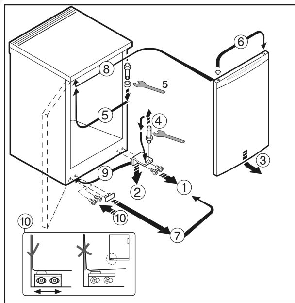
Fig. 6 Ajtófogantyú nélküli berendezések esetén*
