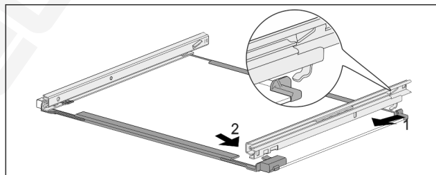
Fig. 45 Üveglap sínnel
