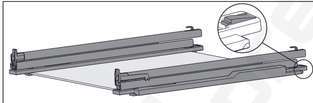
Fig. 48 Üveglap sínekkel és tartóelemekkel
