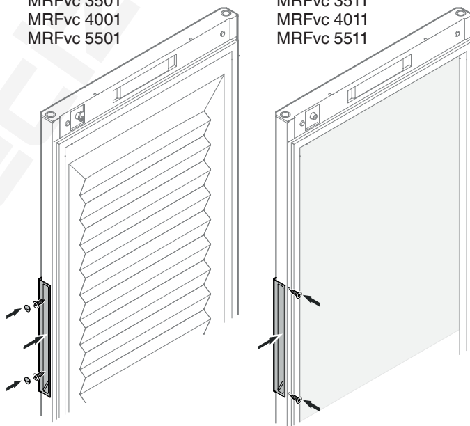
25. Csavarozza fel a fogantyút.
