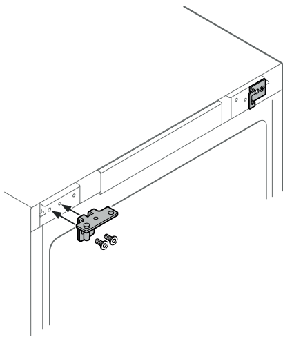
21. Csavarozza fel a csuklópántot.
