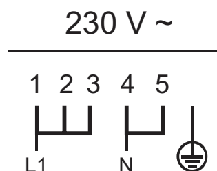
Bekötési rajz
